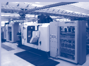
Vertikal-BAZ mit Werkstückspeicher
